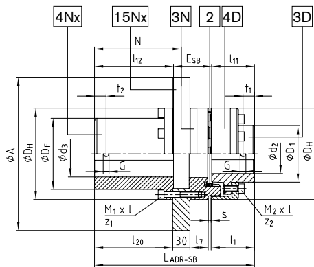
Тип ADR-SB С тормозным диском
